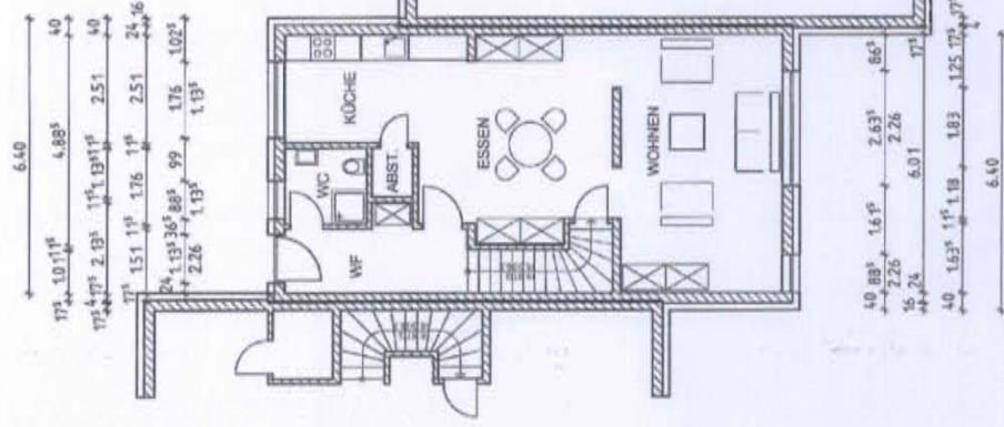
Erdgeschoss
