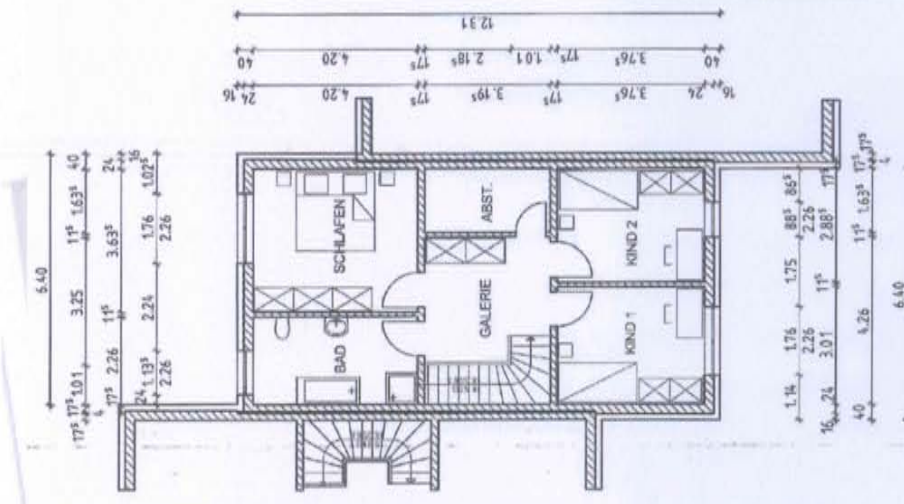
Obergeschoss
